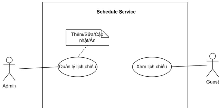
Hình 3.3.1. Usecase diagram Quản lý lịch chiếu
