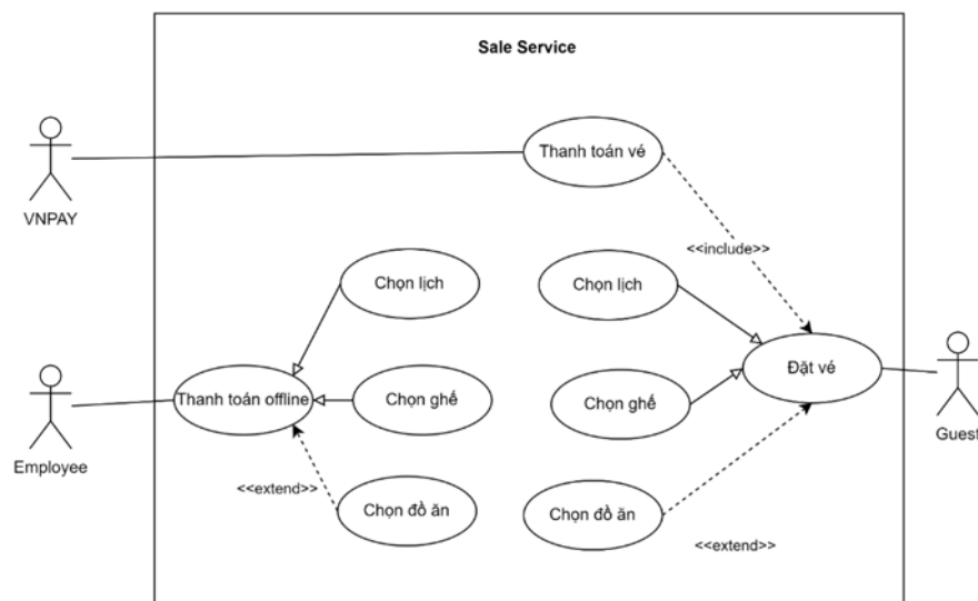
Hình 3.3.2. Usecase diagram Quản lý bán vé
