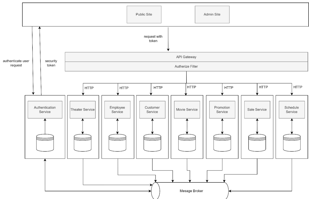
Hình 3.1.1. Kiến trúc toàn bộ hệ thống
