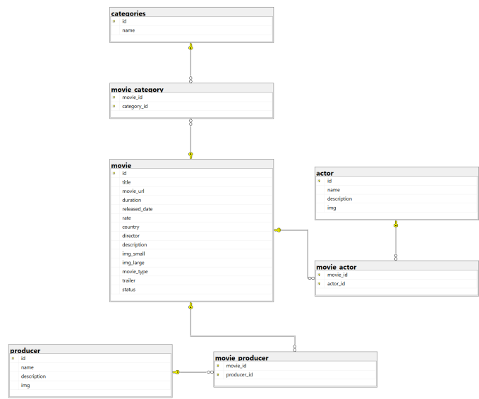
Hình 3.2.7. Cơ sở dữ liệu Movie
