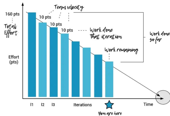
Hình 2.4. Burndown chart
