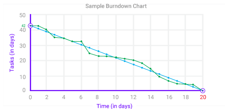
Hình 2.5. Burndown chart (2)
