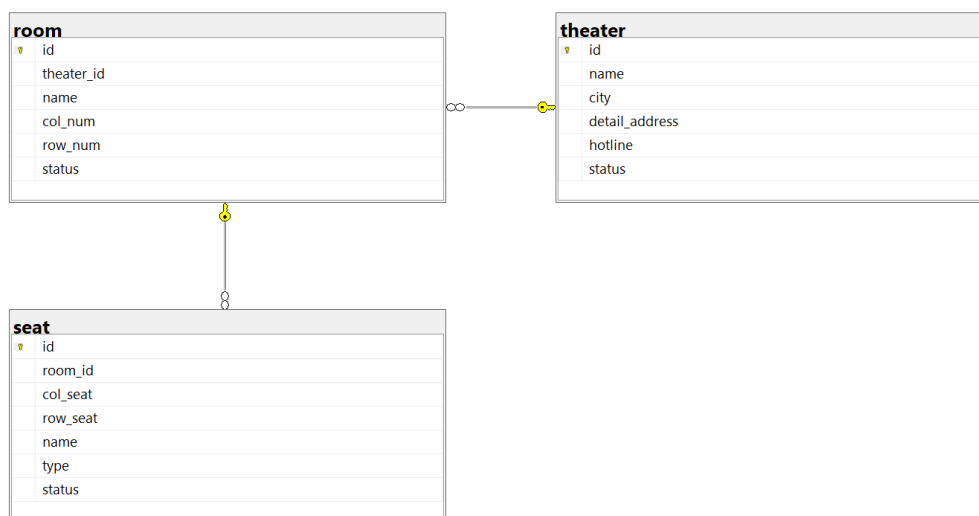
Hình 3.3.4. Cơ sở dữ liệu Theater
