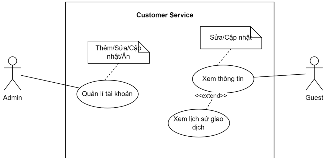
Hình 3.2.4. Biểu đồ use case về quản lý khách hàng
