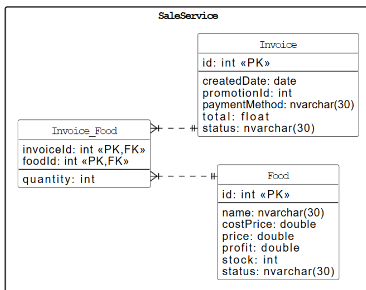
Hình 3.3.5. Cơ sở dữ liệu SaleService
