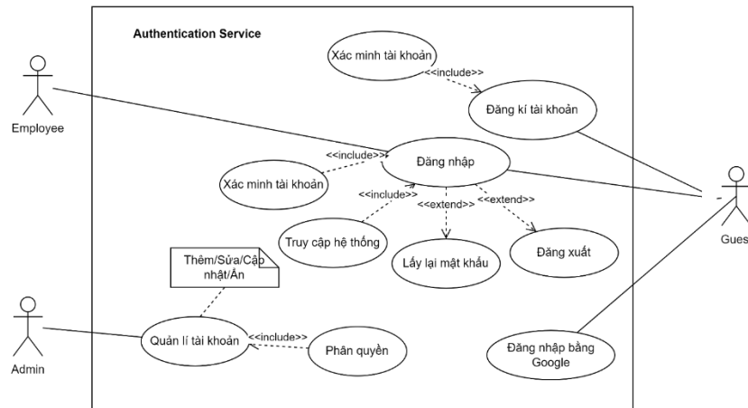
Hình 3.2.1. Biểu đồ usecase Quản lý xác thực người dùng
