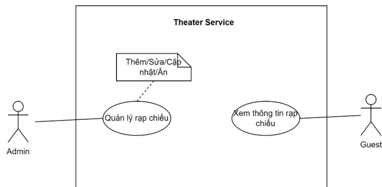
Hình 3.2.3. Biểu đồ use case về quản lý rạp phim
