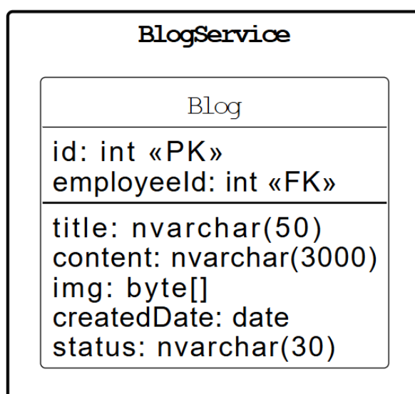
Hình 3.3.6. Cơ sở dữ liệu BlogService
