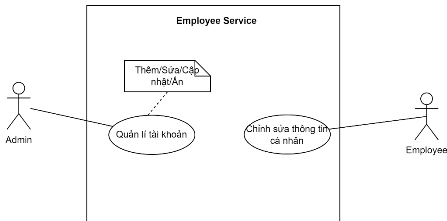
Hình 3.2.5. Biểu đồ use case về quản lý nhân viên
