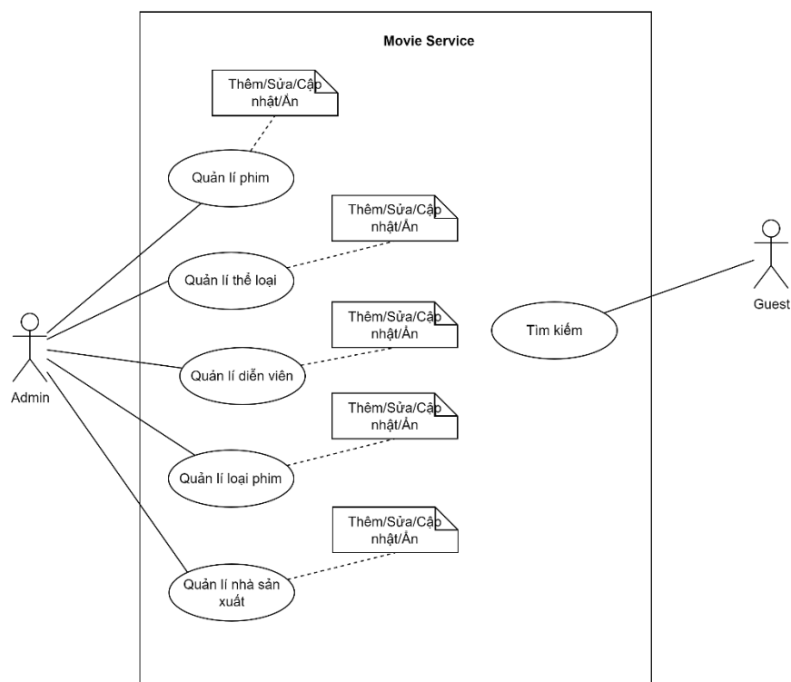
Hình 3.2.2. Biểu đồ use case về quản lý dịch vụ phim
