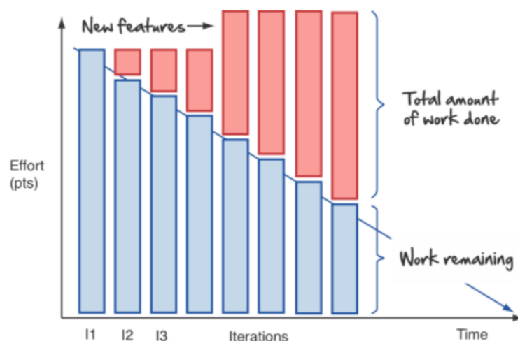
Hình 2.6. Burndown chart (3)
